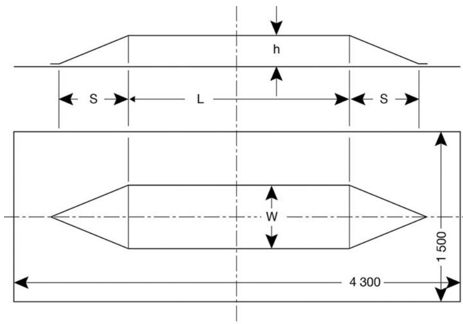
Figura 2 Prova in stripline da 150 mm
