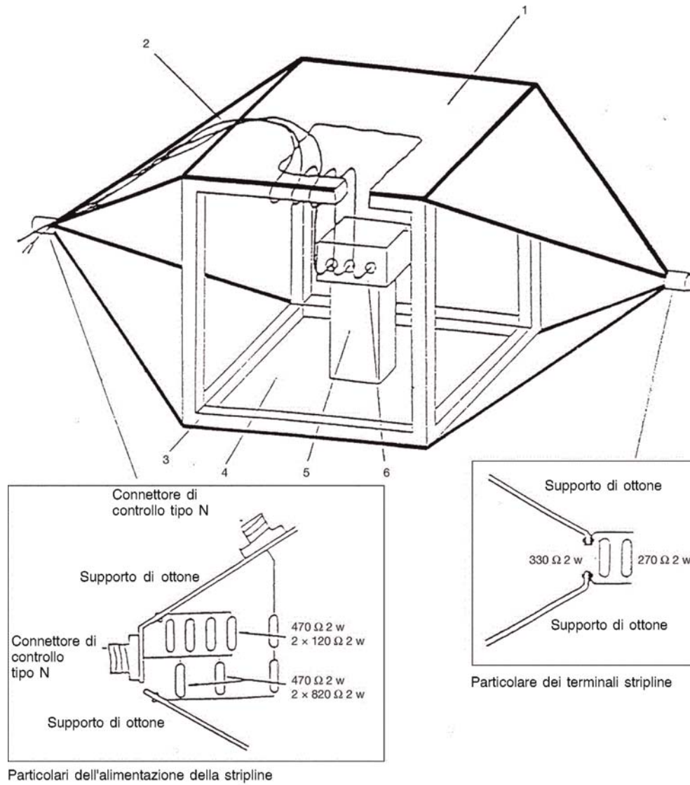
Figura 3 Prova in stripline da 800 mm
